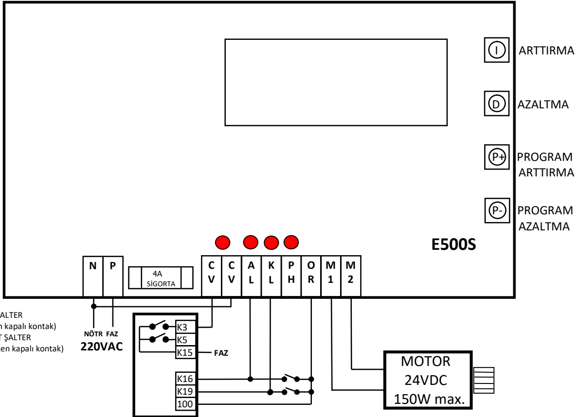
ELEKTRİKSEL BAĞLANTI ŞEMASI - B
