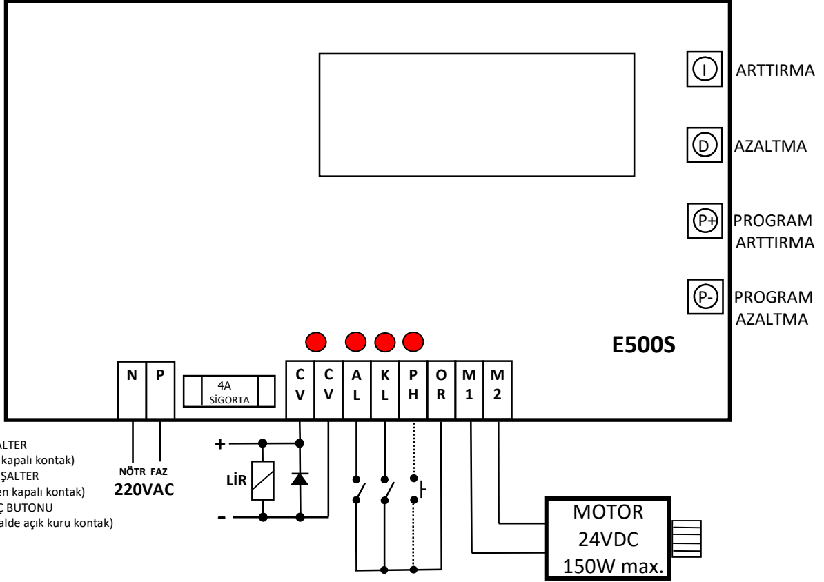
ELEKTRİKSEL BAĞLANTI ŞEMASI - A
