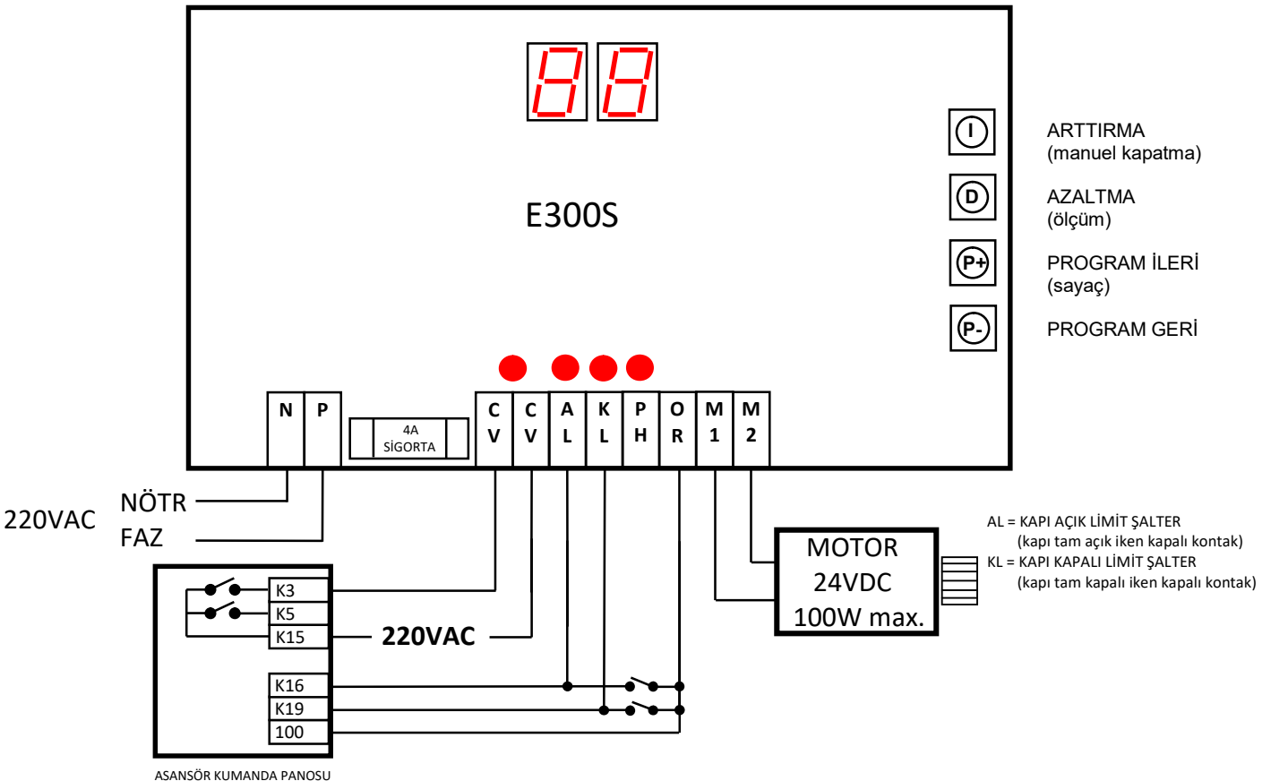
ELEKTRİKSEL BAĞLANTI ŞEMASI - B
