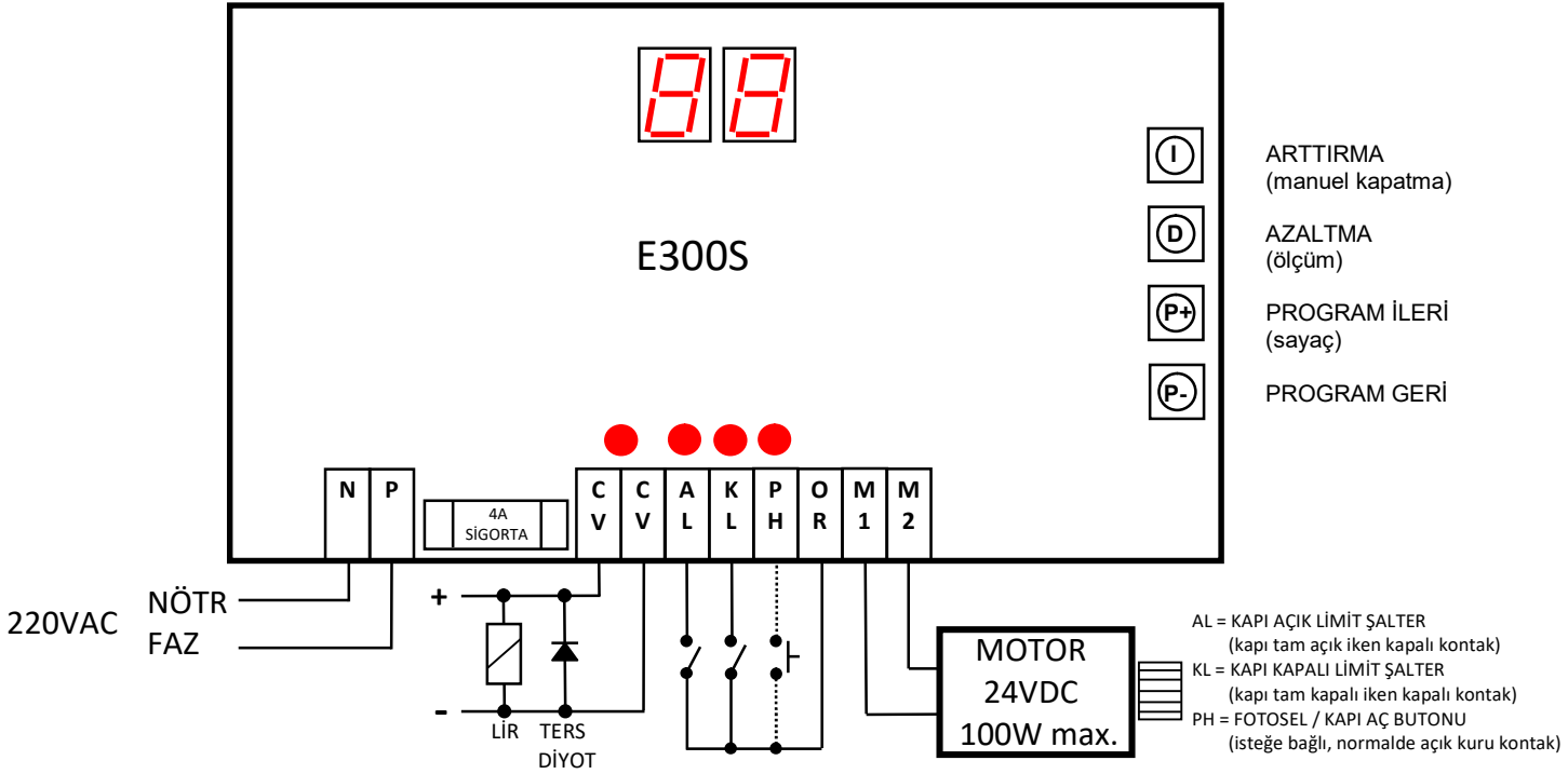
ELEKTRİKSEL BAĞLANTI ŞEMASI - A
